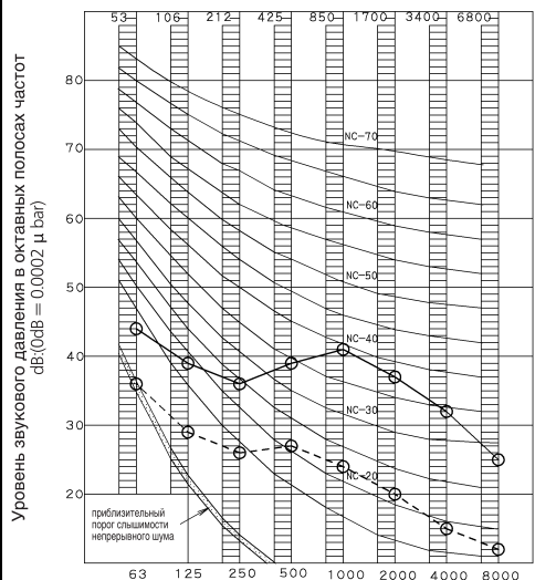
FTXR50E (Охлаждение)
