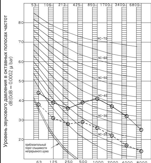
FTXR50E (Обогрев)
