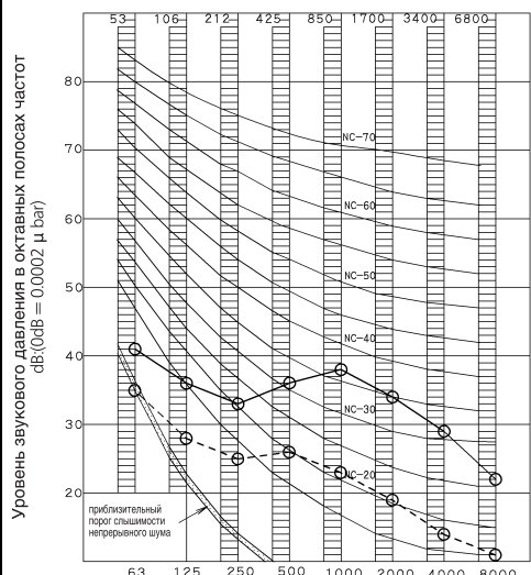
FTXR28E (Обогрев)
