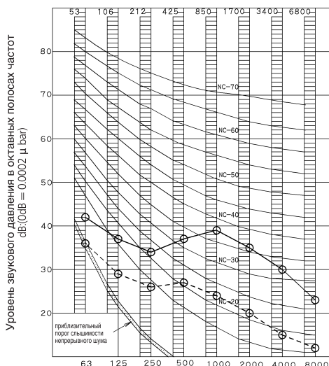
FTXR42E (Обогрев)
