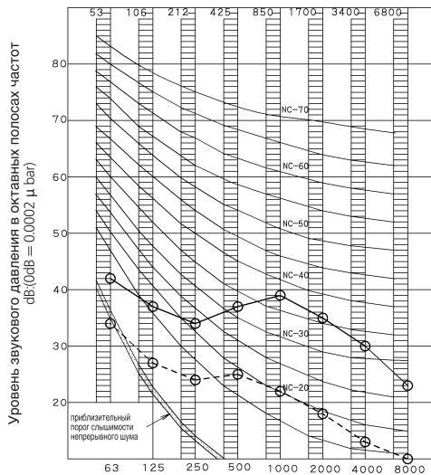
FTXR42E (Охлаждение)
