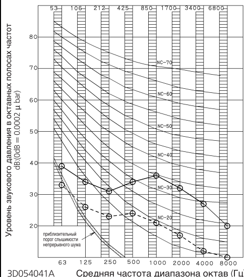
FTXR28E (Охлаждение)
